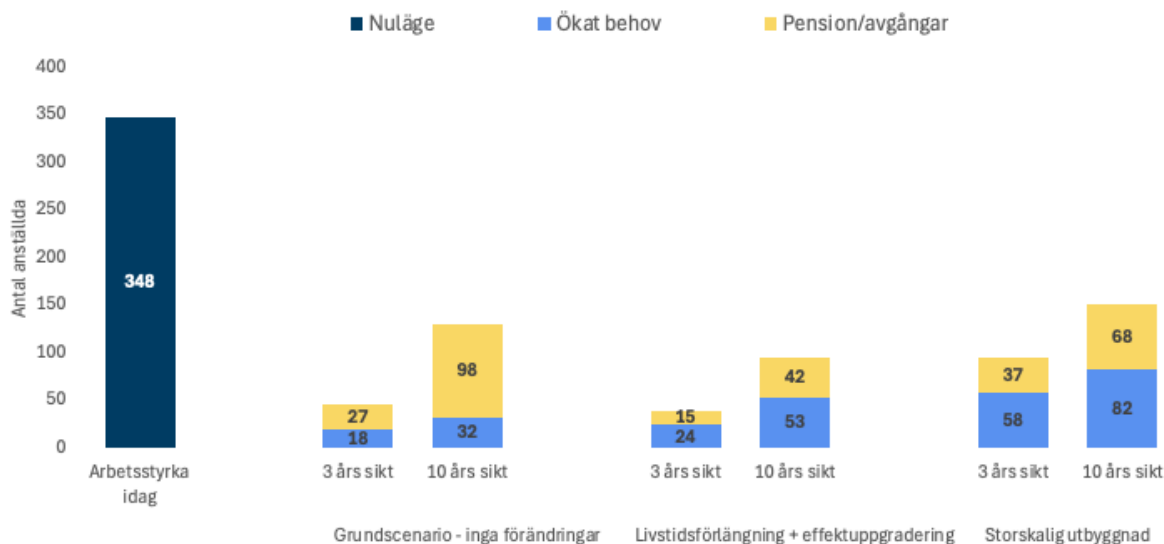
Figur 16: Nuvarande och framtida kompetensbehov inom kärnkraftsteknik, redovisat som heltidsekvivalenter
