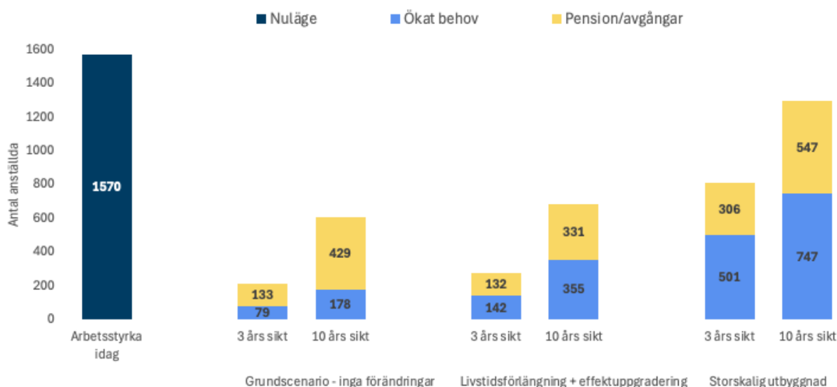
Figur 14: Nuvarande och framtida kompetensbehov inom strålskydd, redovisat som heltidsekvivalenter
