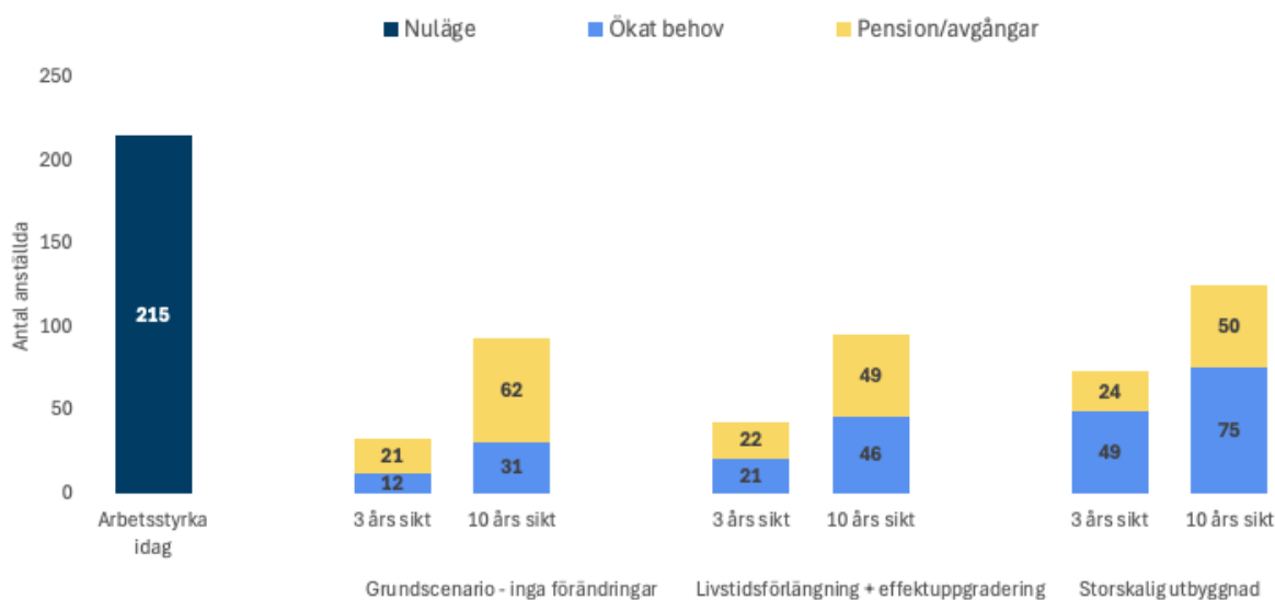
Figur 17: Nuvarande och framtida kompetensbehov inom avfall, redovisat som heltidsekvivalenter
