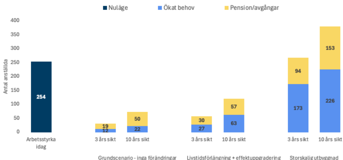
Figur 18: Nuvarande och framtida kompetensbehov inom övrig teknik, redovisat som heltidsekvivalenter
