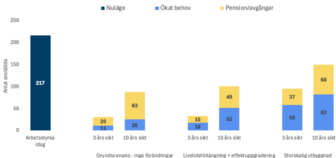
Figur 15: Nuvarande och framtida kompetensbehov inom kemiteknik, redovisat som heltidsekvivalenter
