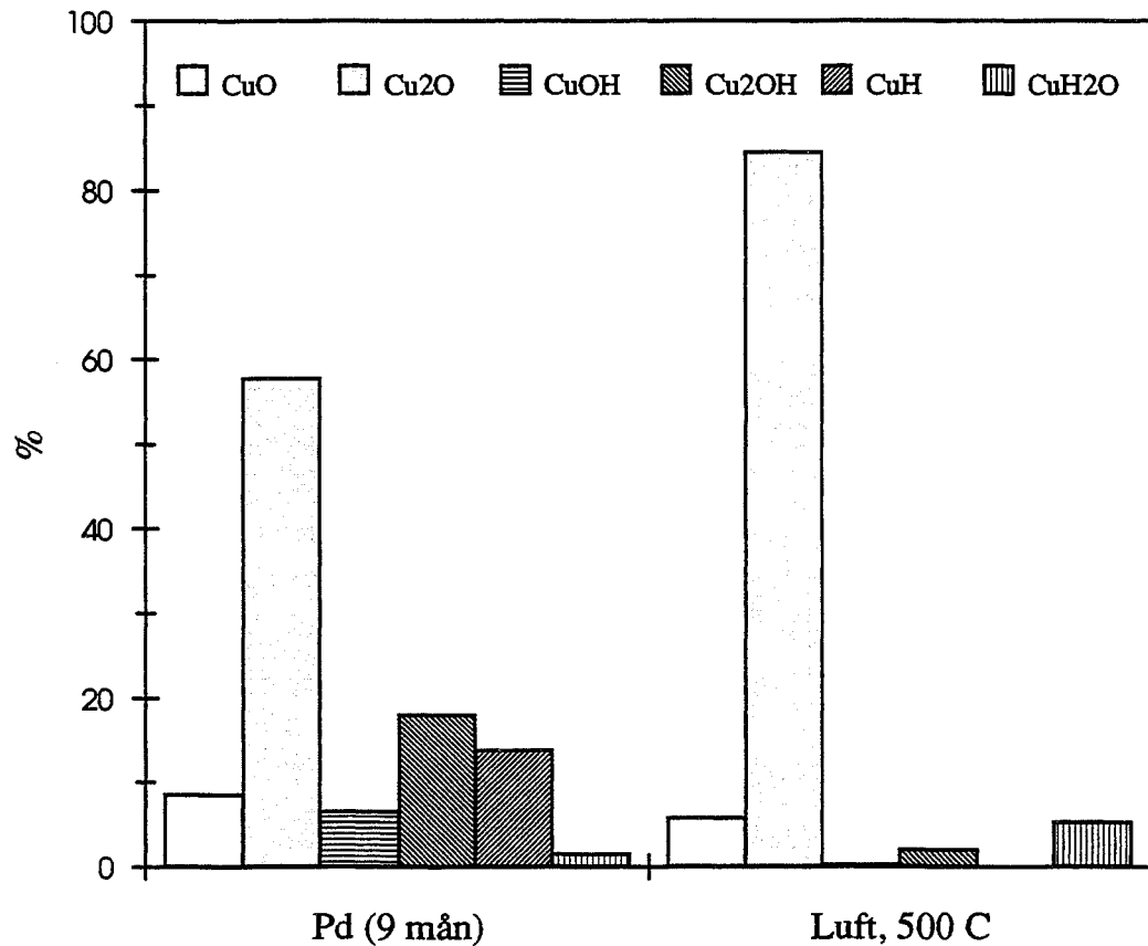
Figur 5. Distribution av olika Cu-O-H fragment vid SIMS-analys av oxidationsprodukter på koppar i Pd-förslutet system vid 50 °C och i luft vid 500 °C
