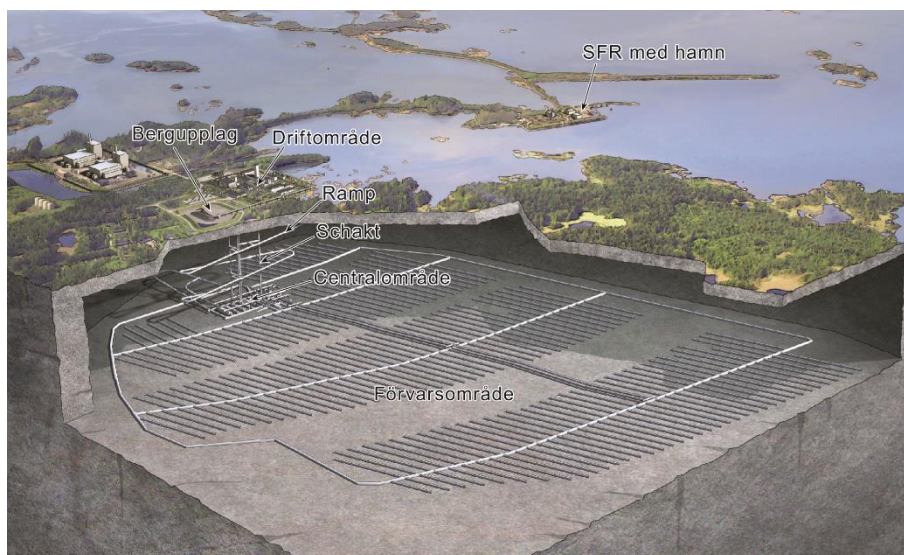
Figur 15. Kärnbränsleförvaret i Forsmark 66 .
