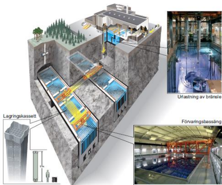
Figur 7. Det centrala mellanlagret för använt kärnbränsle, Clab 42 .
