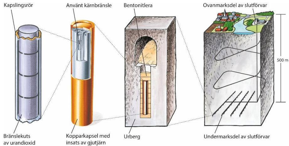
Figur 10. KBS-3 metoden för förvaring av använt kärnbränsle 44
