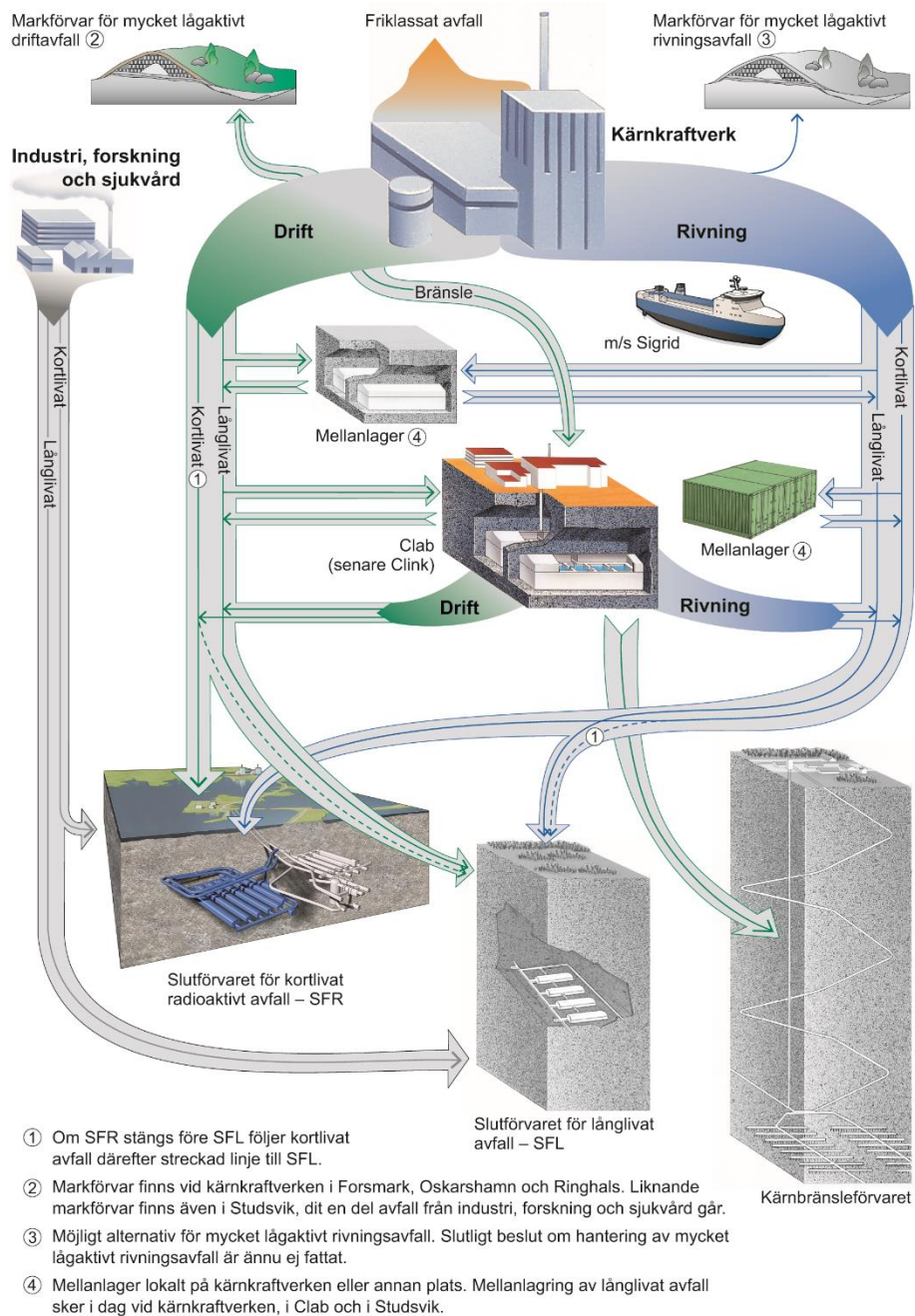
Figur 5. Systemet för att ta hand om Sveriges radioaktiva avfall och använda kärnbränsle. Heldragna linjer representerar transportflöden till befintliga eller planerade anläggningar. Streckade linjer representerar alternativa hanteringsvägar 41 .
