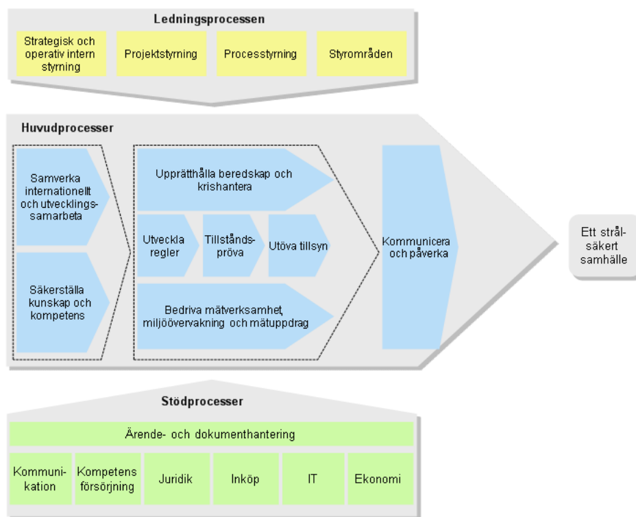
Figur 2. SSM:s huvudprocesser.
