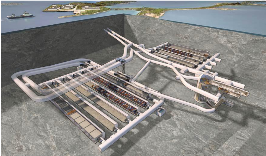
Figur 9. Slutförvar för radioaktivt driftavfall SFR i Forsmark. Till höger den befintliga anläggningen, till vänster den planerade utbyggda delen 43 .
